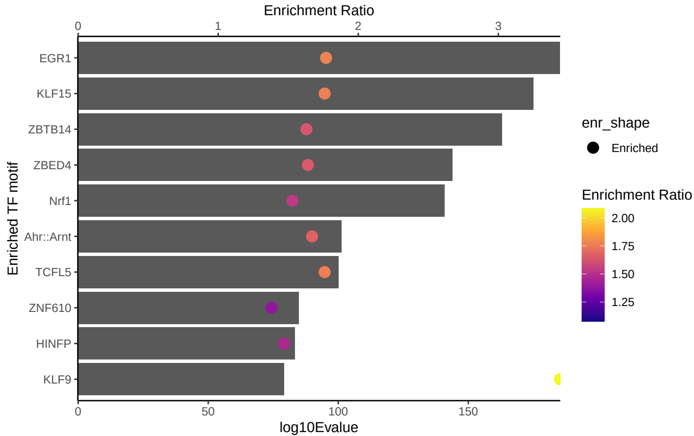
filtered_H3K9me3_Set2_data - 10
